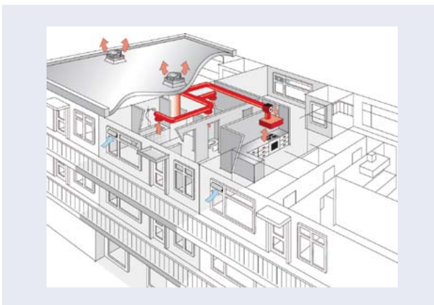
Principetekening collectieve ventilatie in woningbouw
